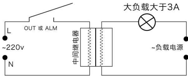
ALM 继电器接中间继电器示意图 注：负载电流大于3A时请用这个接线方式
