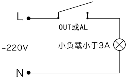
ALM 继电器接负载示意图 注：负载电流要求小于3A
